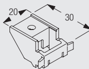
3603 Takfäste
