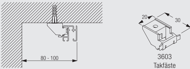
3603 Takfäste
